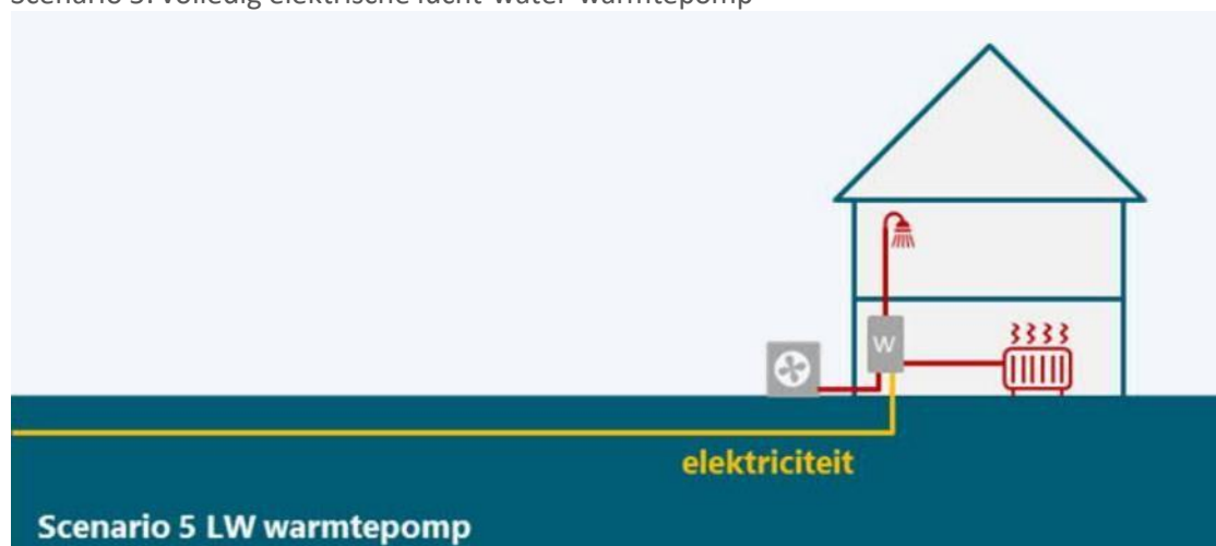
Scenario 5: volledig elektrische lucht-water-warmtepomp
